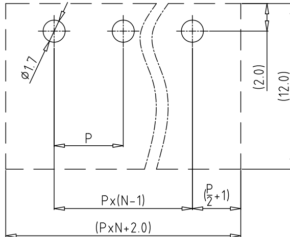
Remmended P.C.B Layout
