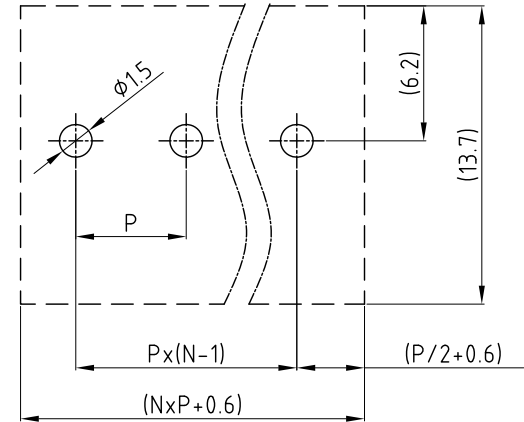
Remmended P.C.B Layout
